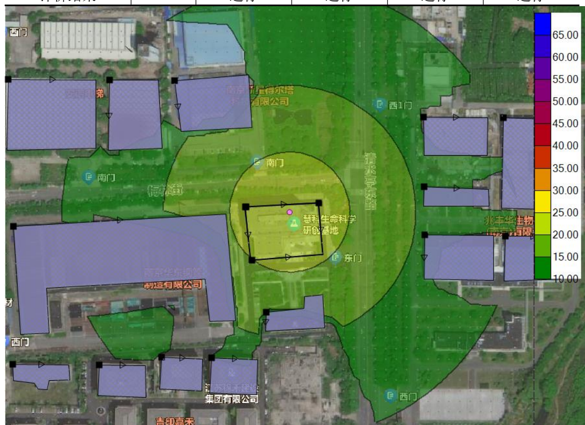
图 4-4 噪声 (昼间) 贡献值预测图
