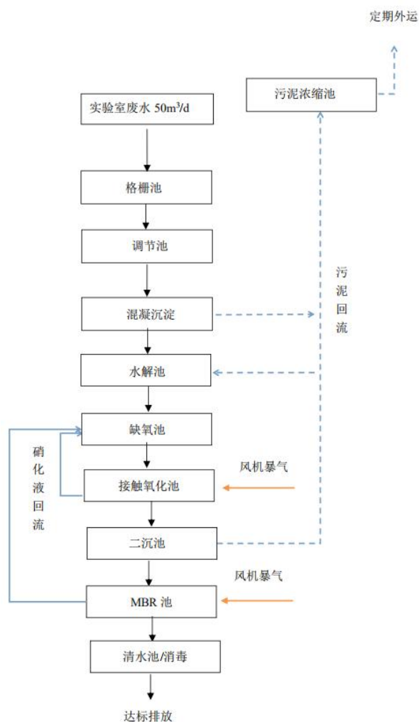
图 4-2 慧科污水处理站工艺流程示意图
