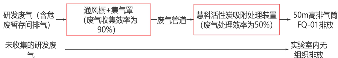
图 4-1 废气收集、处理示意图
