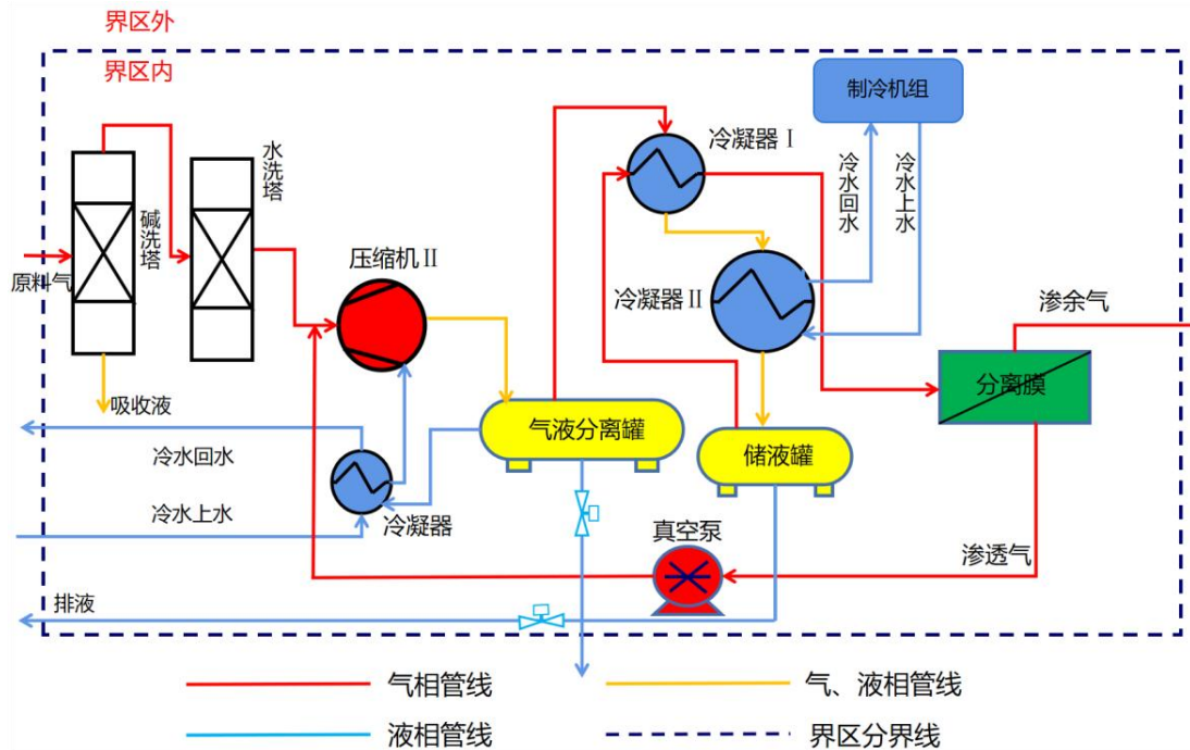
图 6.2-1 工艺流程简图
