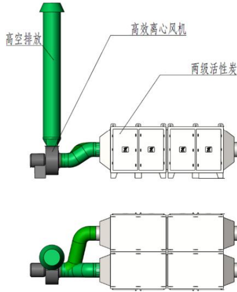
图6.2-3 二级活性炭装置结构示意图
