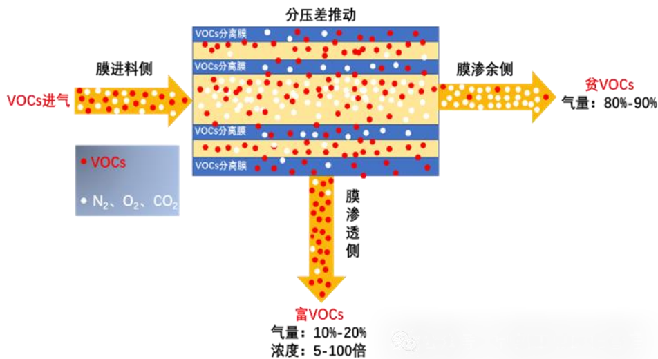
图 6.2-2 膜分离工作原理图
