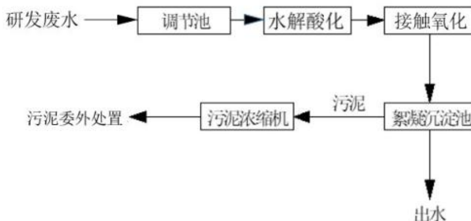
图 4-2 聚慧园污水处理站污水处理工艺流程图
