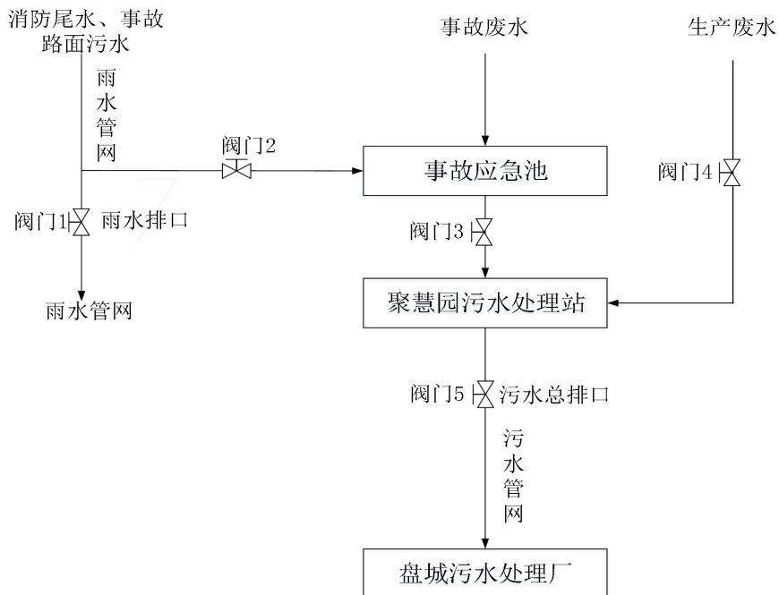
图 4-4 防止事故废水进入外环境的控制、封堵系统图
