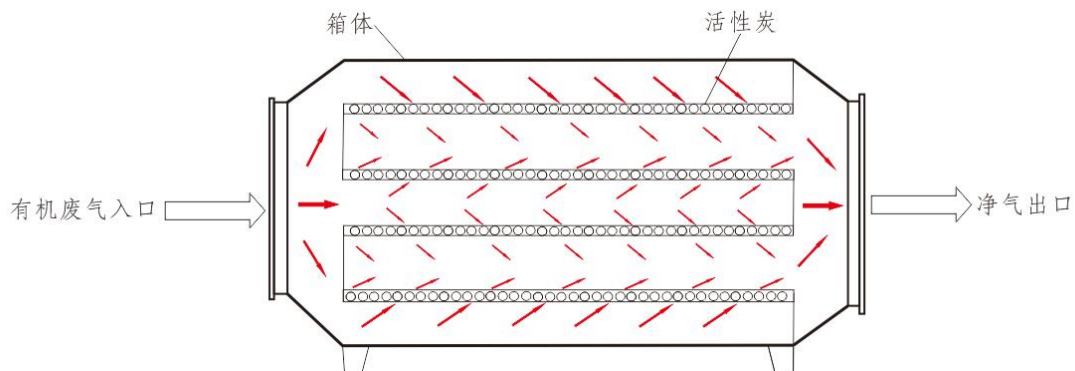
图 4-2 活性炭吸附塔结构示意图
