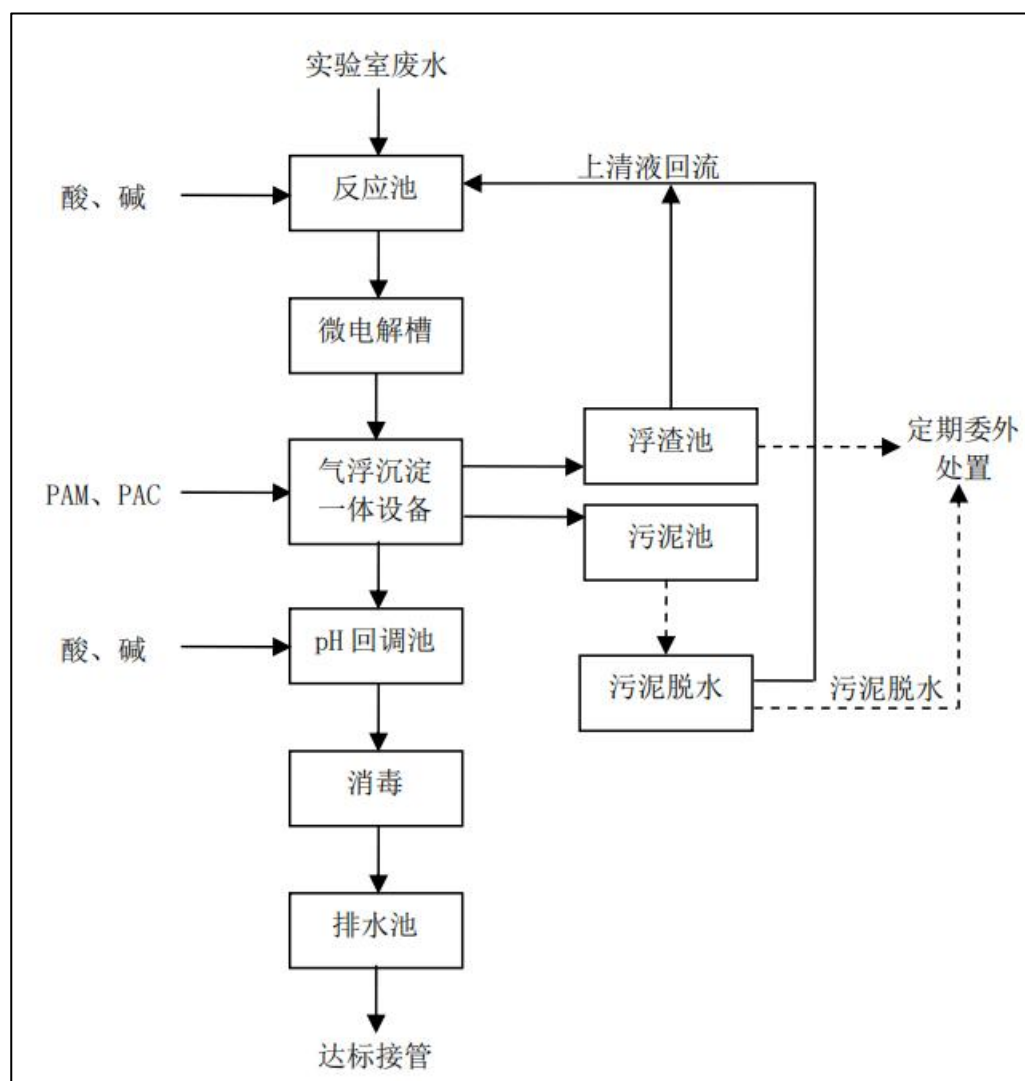
图 4-1 慧科园区污水处理站废水处理工艺流程图
