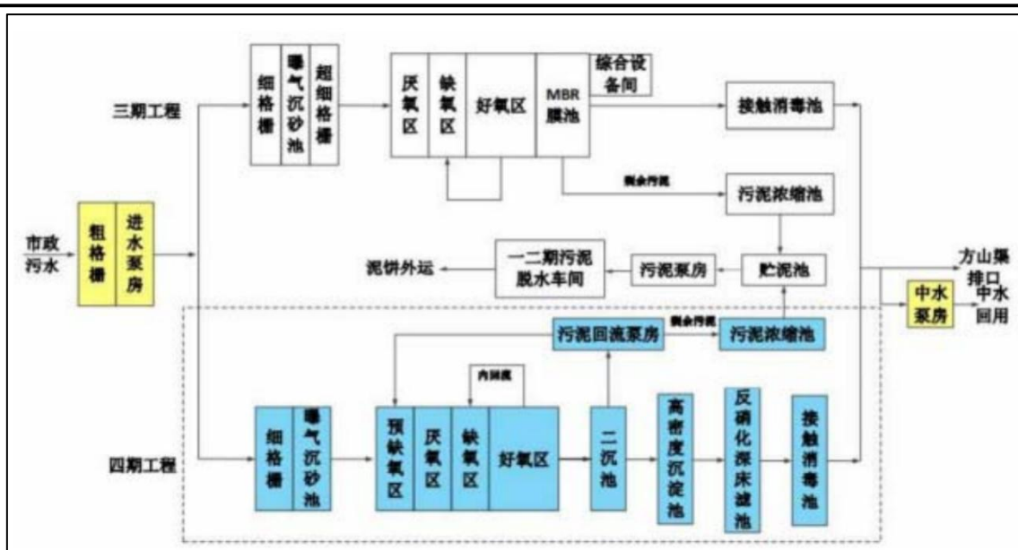
图 4-2 江宁科学园污水处理厂三期工艺流程图
