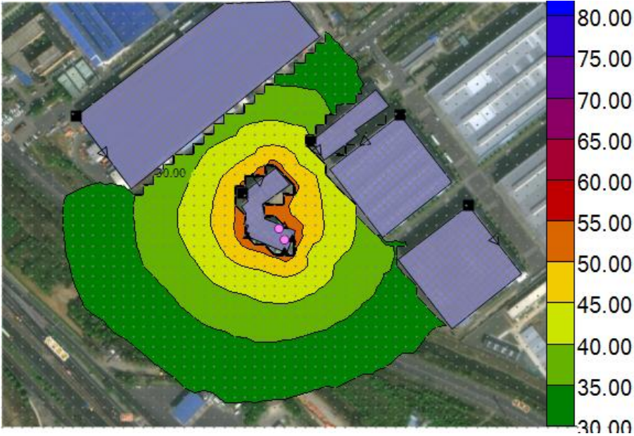
图 4-3 企业厂界噪声预测结果等值线图
