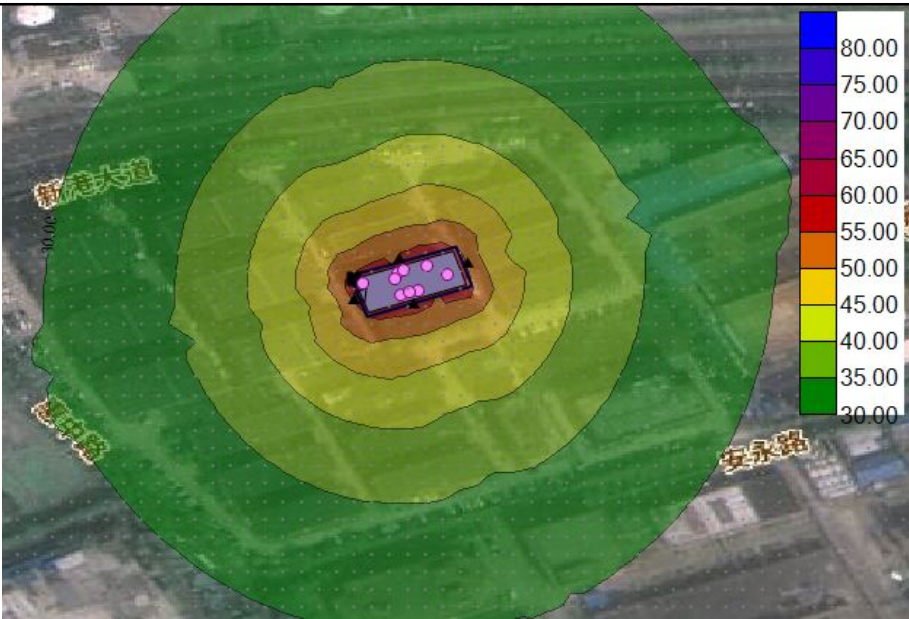
图 4-3 厂界噪声预测图
