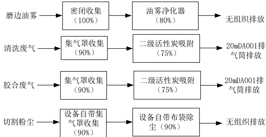
图4-1 本项目废气收集处理工艺流程图
