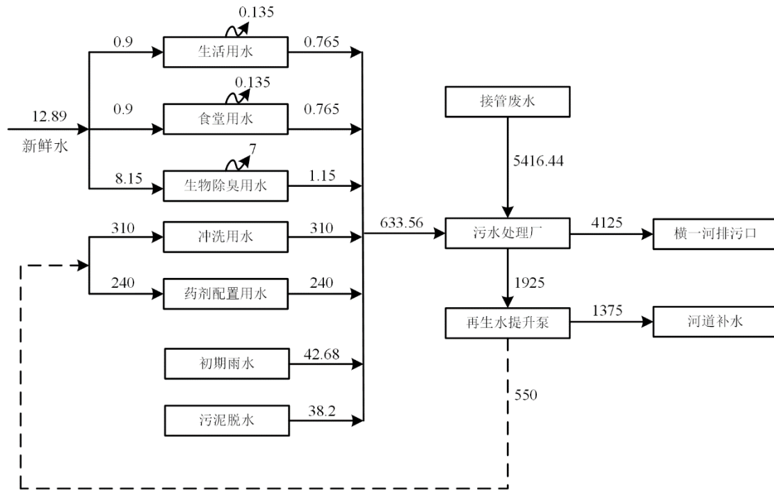
图 3.3-2 项目水平衡图 (m³/d)
