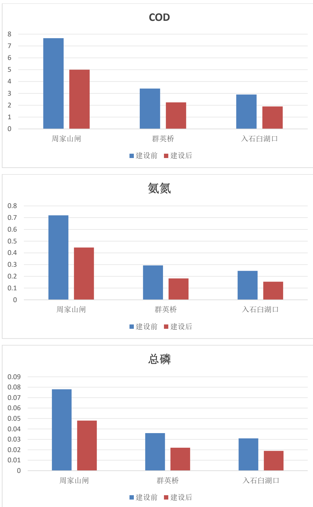
图 5.2-2 枯水期项目建设前后对重要断面水质影响结果
