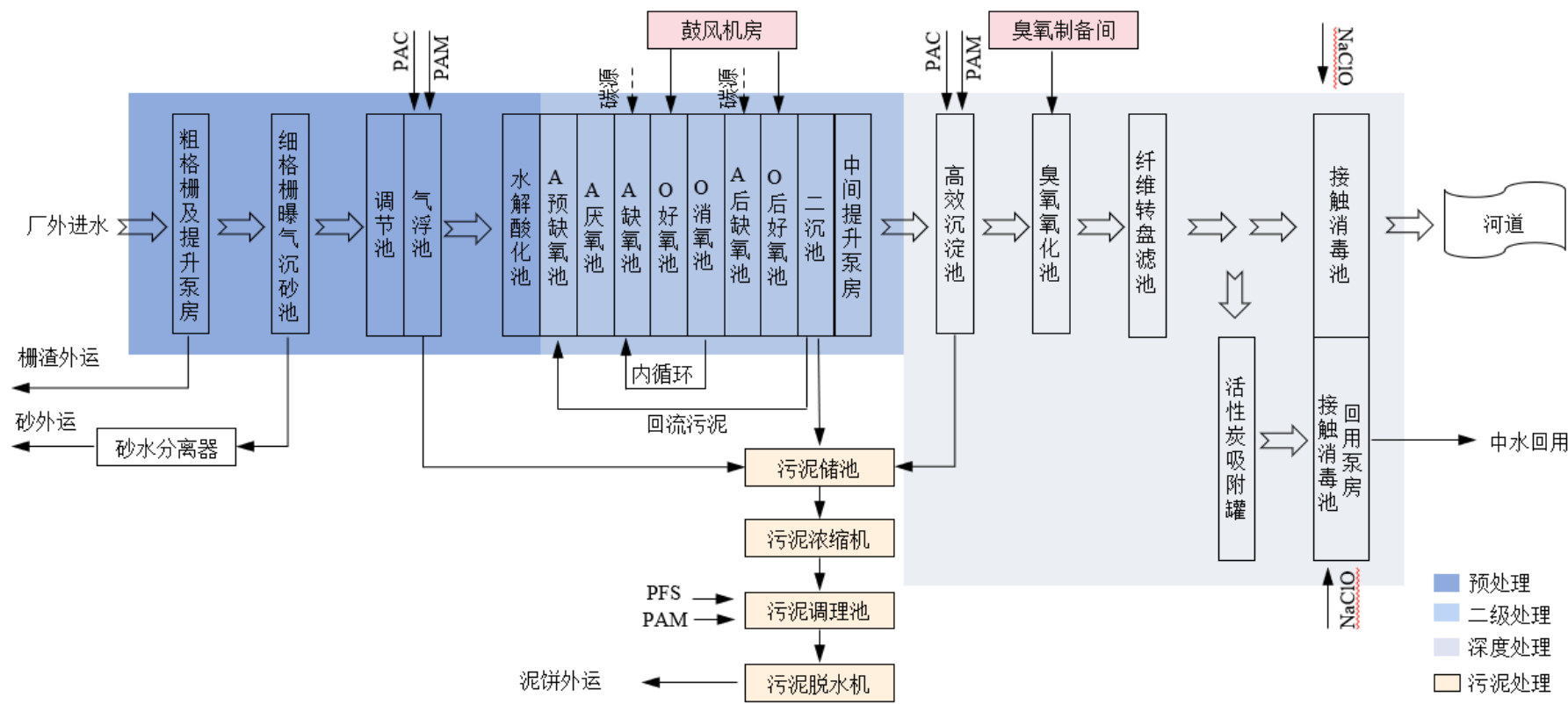
图 3.1-6 工业废水处理中心工艺流程图
