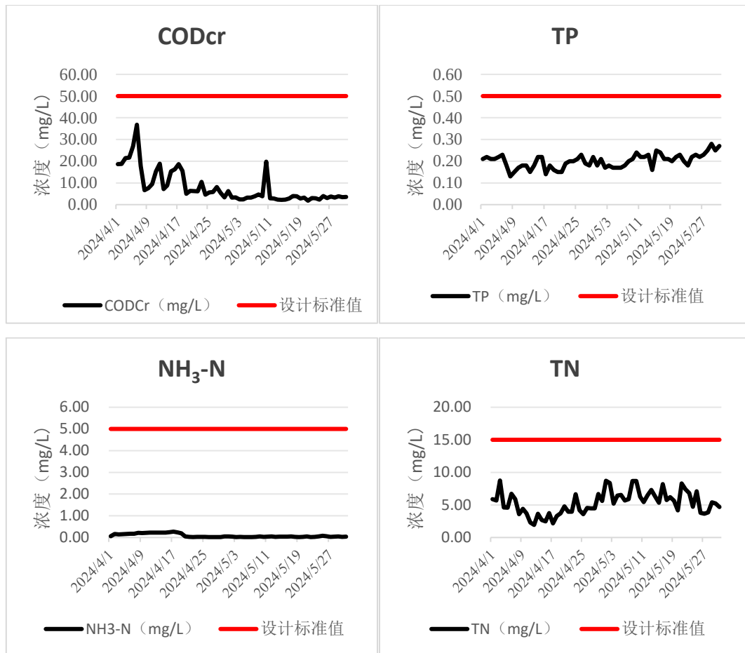
图 3.1-4 白马污水净化站监测出水水质变化图
