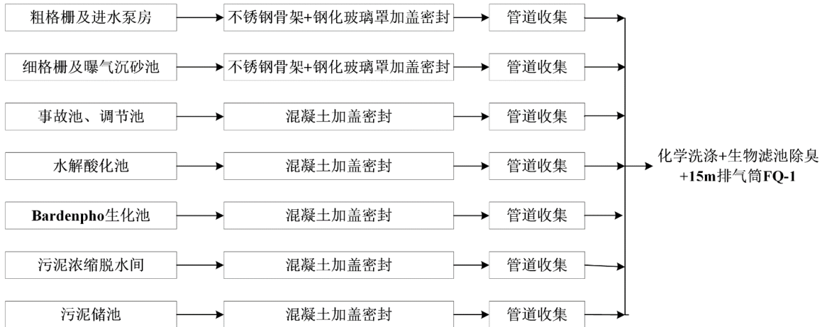
图 6.1-1 有组织废气产生、收集、处理情况示意图
