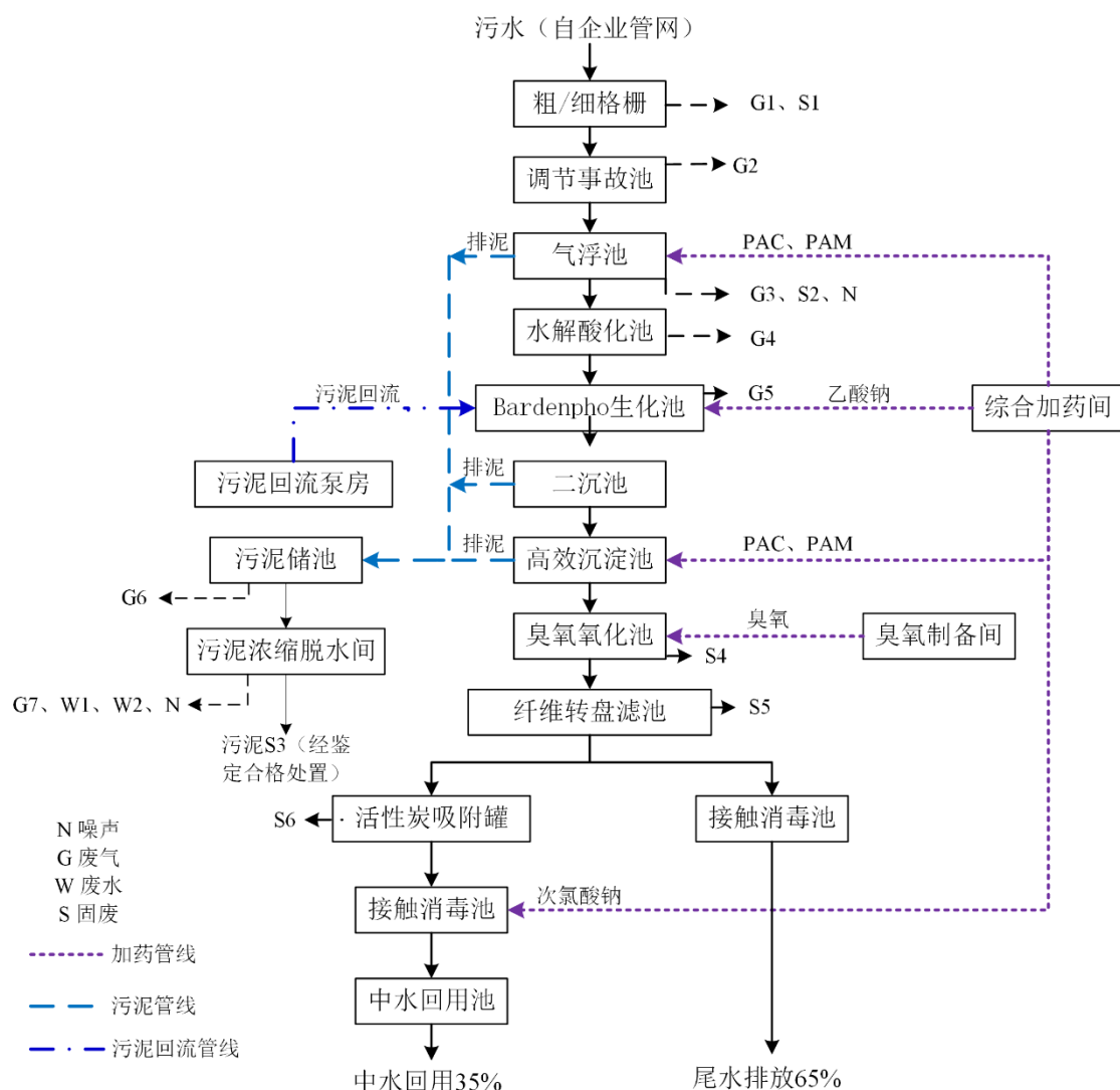
图 3.2-1 污水处理工艺流程及产污环节示意图
