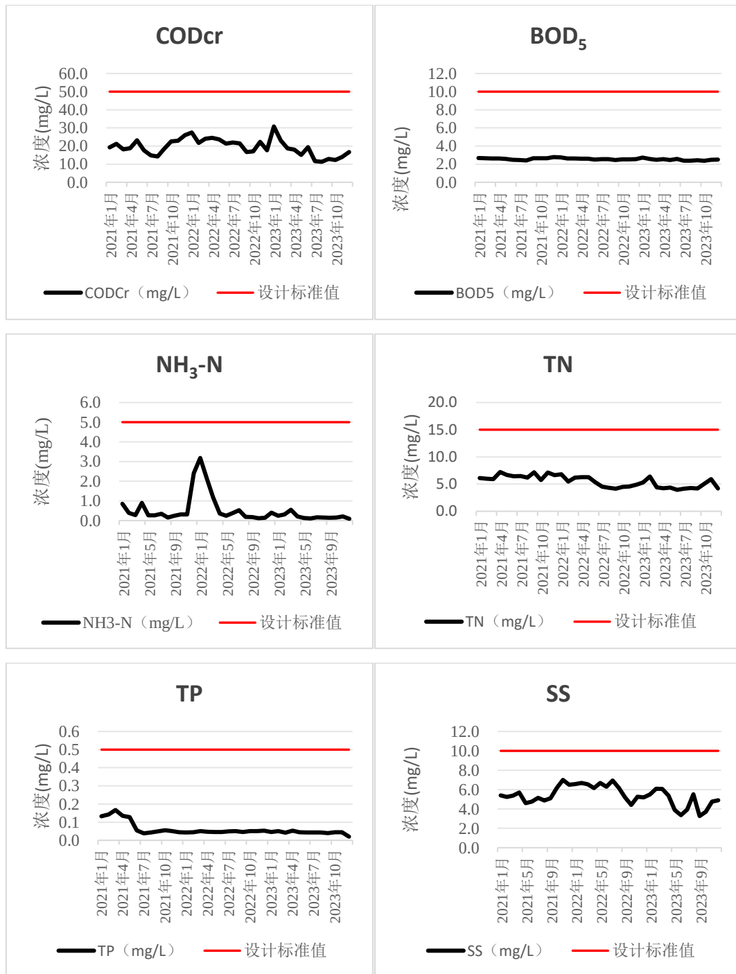
图 3.1-3 2021~2023 年白马污水处理厂逐月监测出水水质变化图
