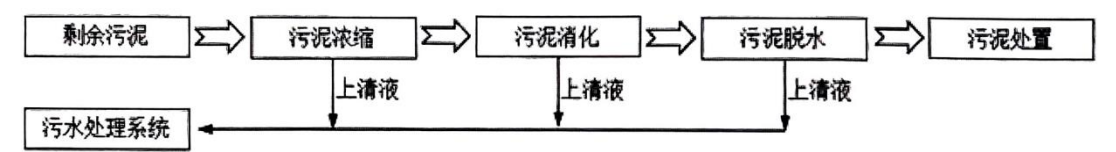
图 3.1-8 典型污泥处理工艺流程图
