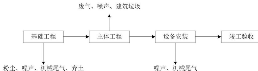
图 3.3-1 污水处理厂施工期流程及产排污节点
