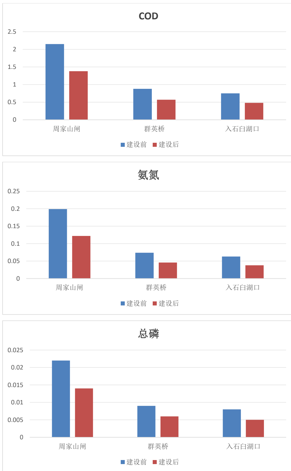
图 5.2-3 丰水期项目建设前后对重要断面水质影响结果
