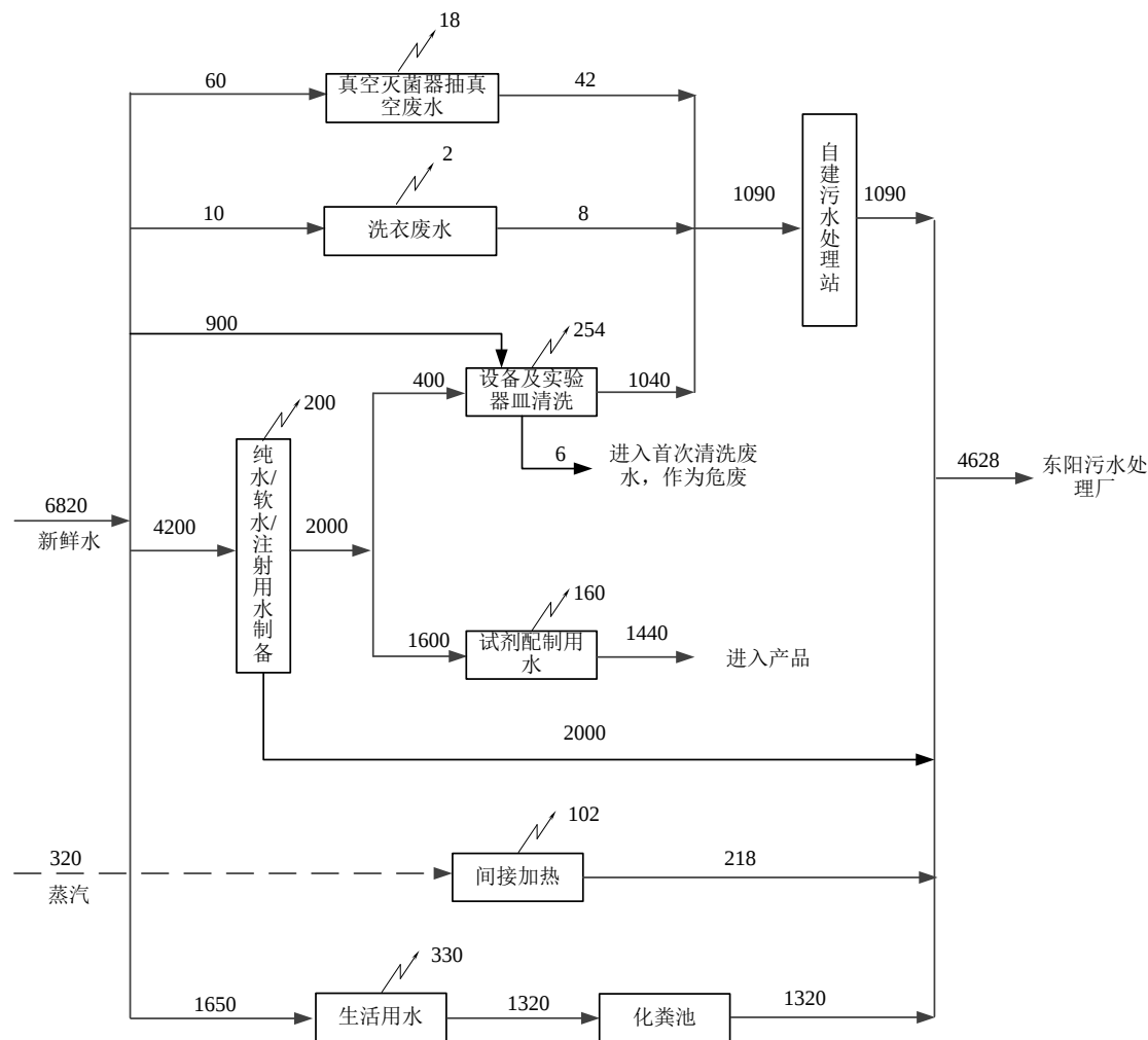
图 2-1 项目实际用水平衡图（单位：m³/a）
