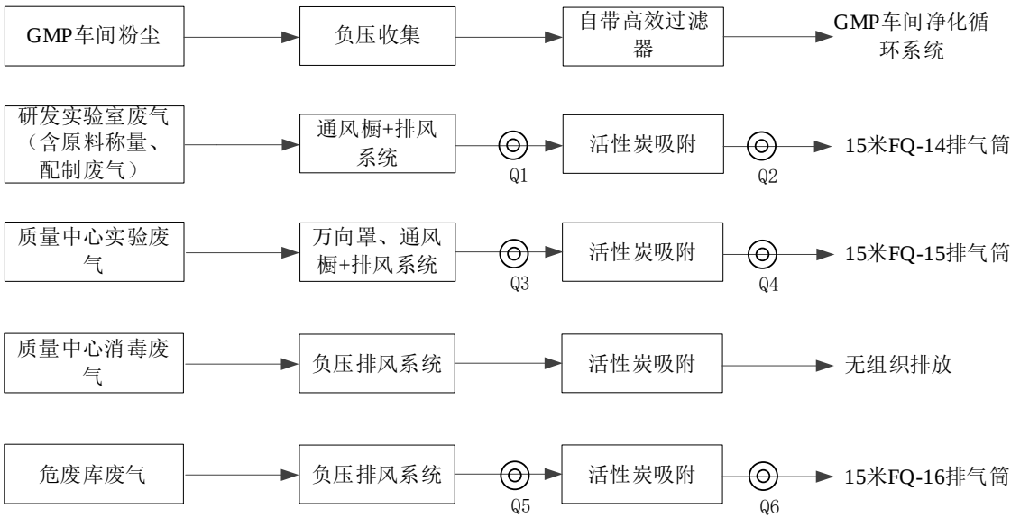
图 3-3 废气收集处理示意图
