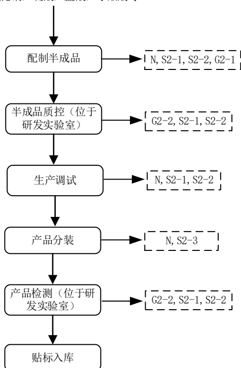
图 2-3 工艺流程及产污环节图
