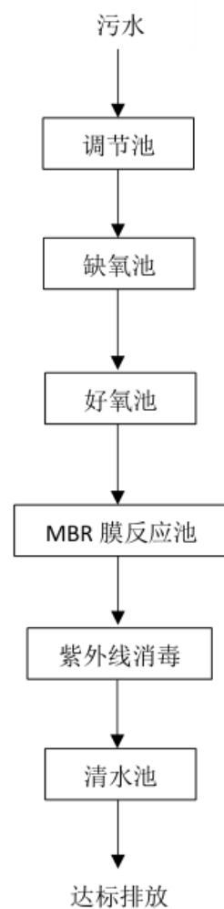
图 3-1 企业自建污水处理设施工艺流程图
