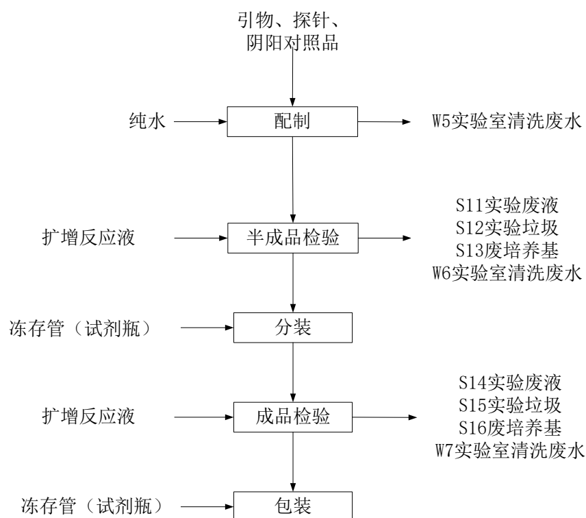
图 2-3 核酸扩增试剂盒生产工艺流程图
