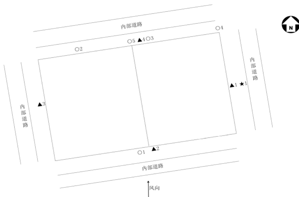
图 3-6 无组织废气、废水及噪声监测点位示意图（2022.4.28、2022.4.29）
