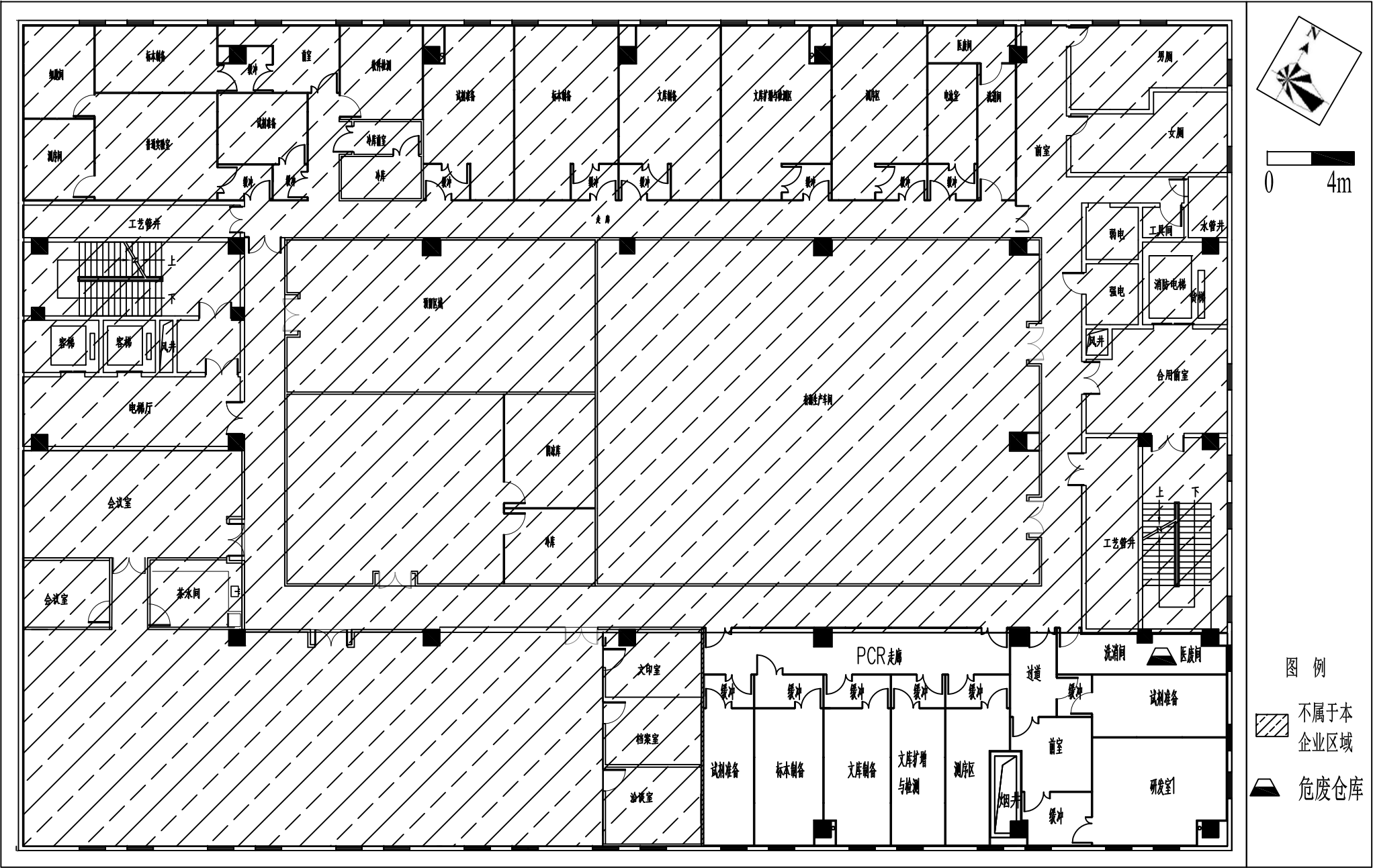
附图3-1 建设项目B栋2F平面布置图
